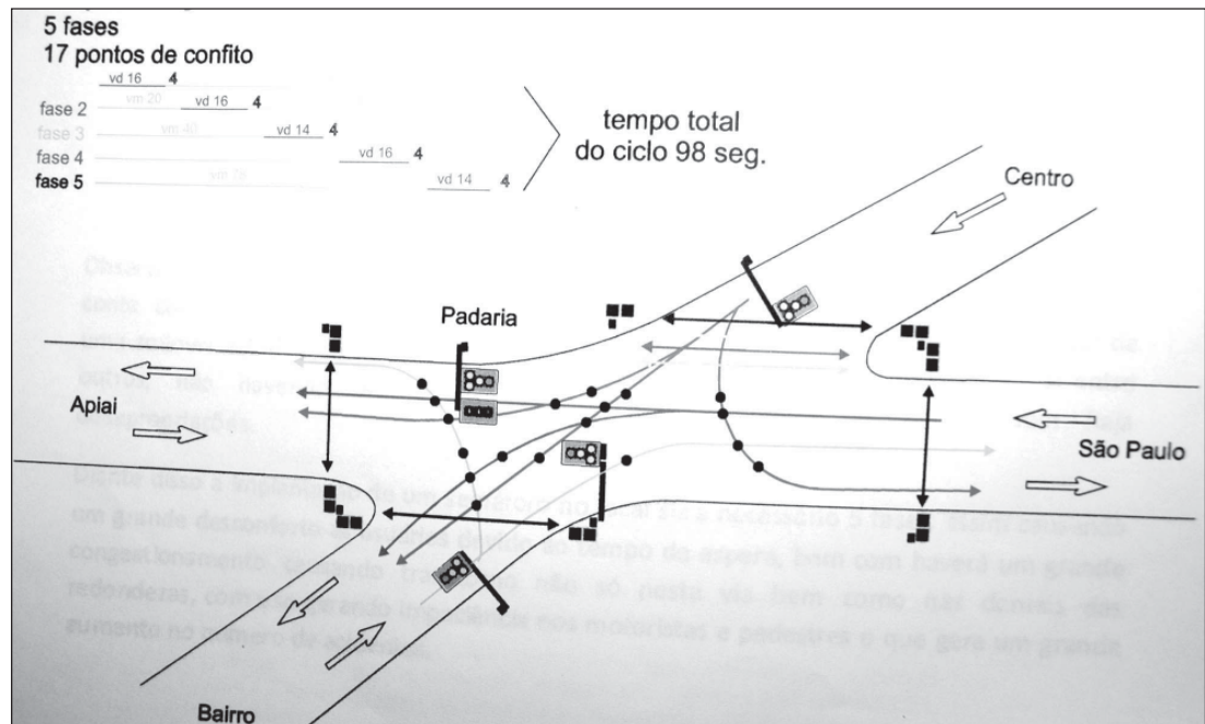
Esboço técnico do projeto para corrigir pontos críticos da avenida
